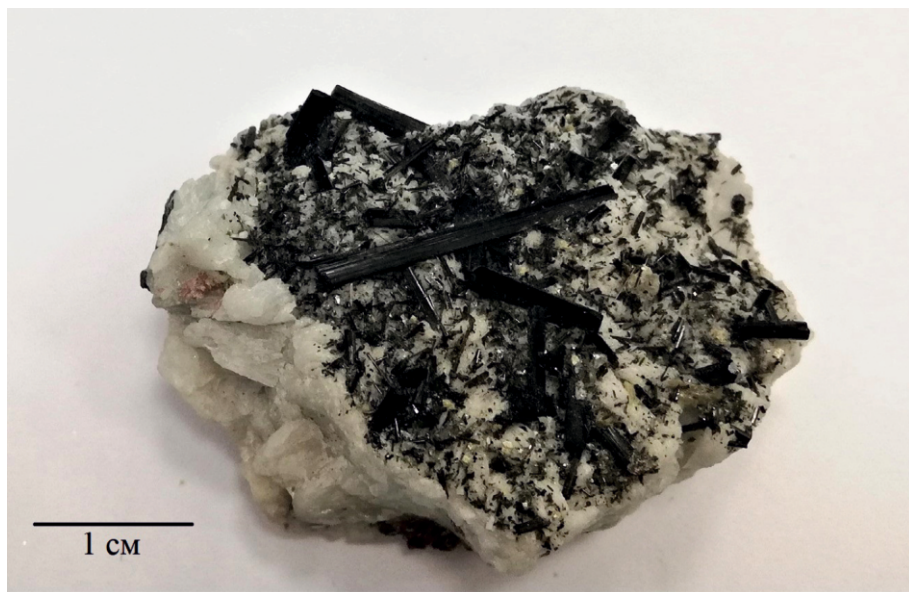
Рис. 2. Шерл. Копь Казенница. Обр. 5. Фото Т.А. Гвозденко
