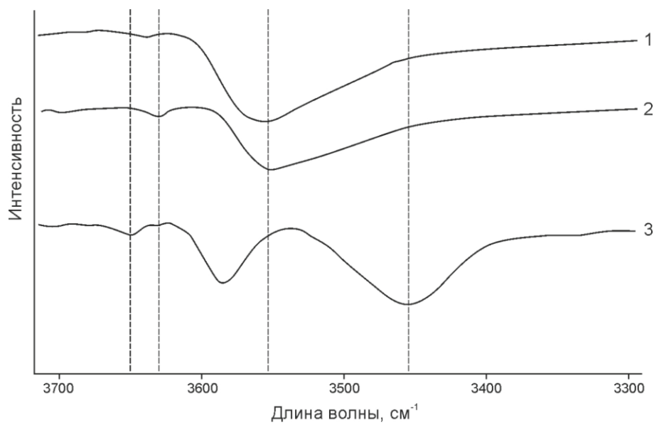
Рис. 5. ИК спектры образцов турмалинов: 1 – дравит, копь Буженинов Бор. Обр. 64.2; 2 – шерл, копь Министерская. Обр. 48; 3 – эльбаит, Липовка. ГГМ РАН. Инв. МН-33793
